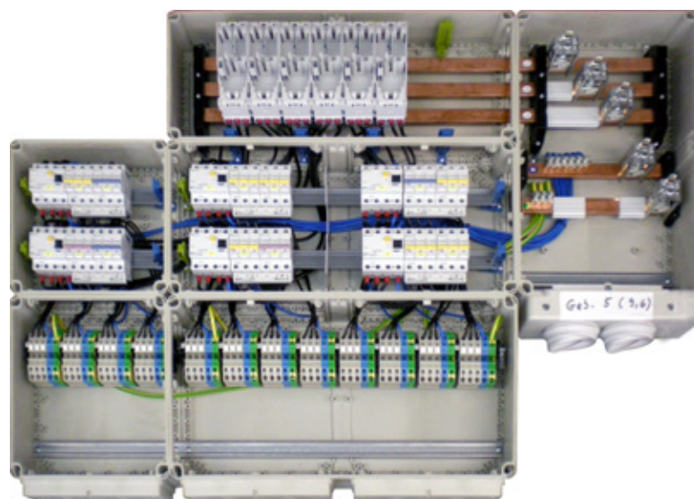
Nennstrom 250A
